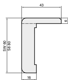
Rohový prvok zárubne SW, S8 obložka standard
