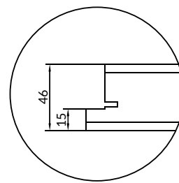
Rez dverí (hrúbka 46mm)
