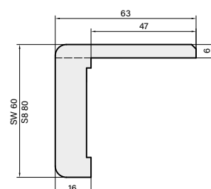
Rohový prvok zárubne SW, S8 predĺžená obložka o 2 cm
