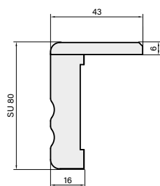
Rohový prvok zárubne SU obložka standard
